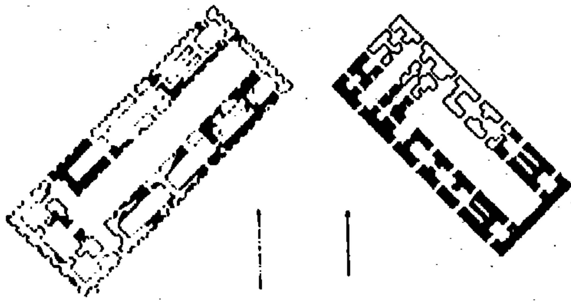
شكل (٩٠) معبدا إنانا في اوروك الأول من الطبقة السادسة ٣٢٠٠ ق.م الثاني من الطبقة الخامسة ٣٤٠٠ ق.م ( المعبد الصخري )
